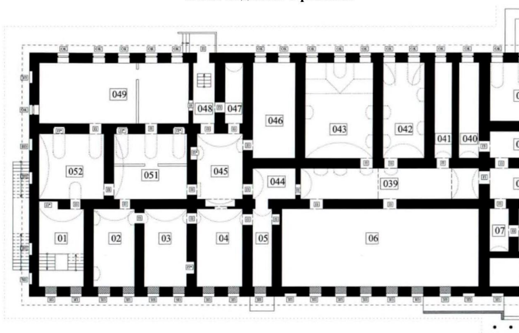
План подвала. Фрагмент
