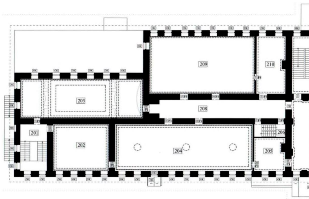
План второго этажа. Фрагмент
